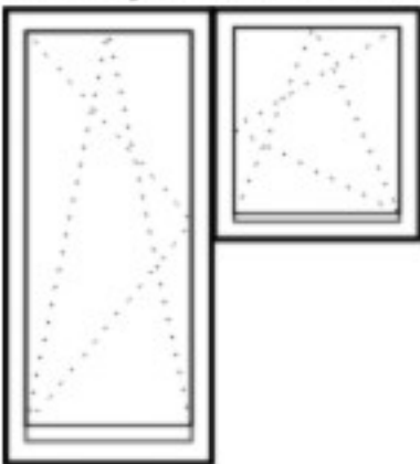
13 - sestava - balkónové dveře + jednokřídlé okno
